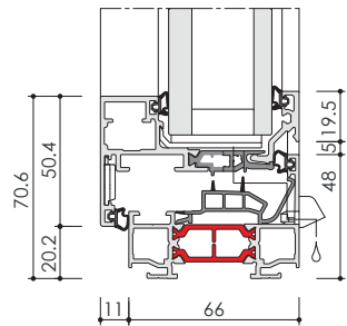
➤ INFINEO CAGE À TÔLE
