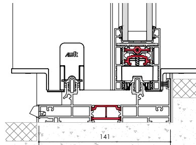
› INFINEO SEUIL STANDARD SUR 2 RAILS
