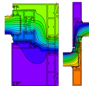
› INFINEO NOEUD THERMIQUE
