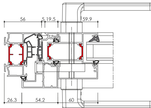
➤ INFINEO CÔTÉ SERRURE 1 VANTAIL
