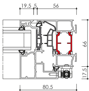
➤ INFINEO CAGE À TÔLE
