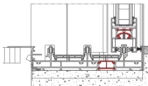
› INFINEO SEUIL INTÉGRÉ - DORMANT 3 RAILS
