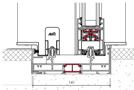
› INFINEO SEUIL INTÉGRÉ - DORMANT 2 RAILS
