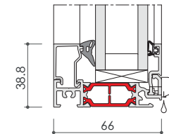
➤ INFINEO SEUIL PMR DÉTAIL 1
