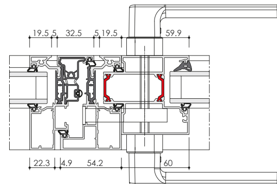
➤ INFINEO MONTANT LATÉRAL
