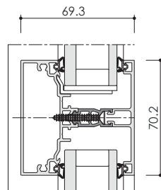
➤ INFINEO TRAVERSE INTERMÉDIAIRE
