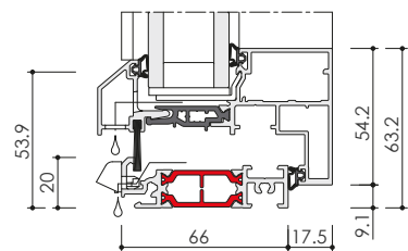
➤ INFINEO SEUIL PMR
