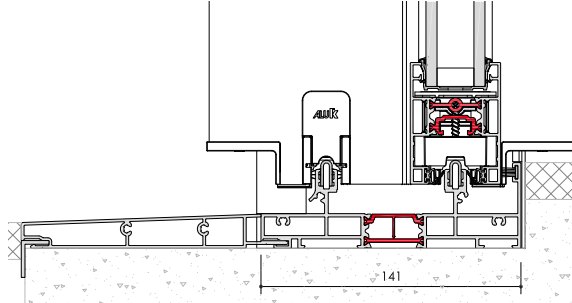
› INFINEO SEUIL GALANDAGE
