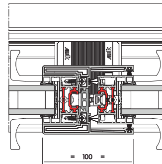
› INFINEO NOEUD CENTRAL 4 VANTAUX
