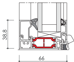
➤ INFINEO SEUIL PMR DÉTAIL 2
